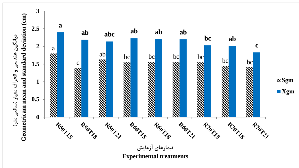
شکل ۴- اثر سرعت مارپیچ و زمان بر شاخص‌های خرد شدن مواد مخلوط (کل الک‌ها)
