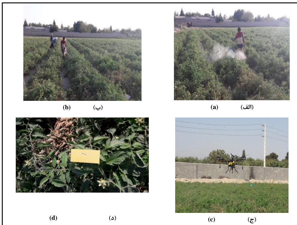
شکل ۱- روش‌های مختلف سمپاشی: الف) سمپاش لانس‌دار، ب) سمپاش اتومایزر، ج) پمپاد سمپاش و د) تعیین یکنواختی پاشش به کمک کارت حساس
