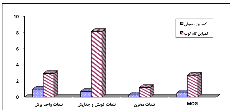
شکل ۳- مقایسه تلفات کمباین معمولی و کاه کوب کلاس
